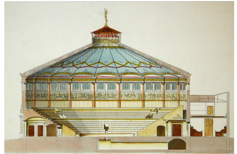
Jacques-Ignace HITTORFF, Cirque Napoléon (Cirque d'Hiver) 11 décembre 1852 42 m de diamètre
